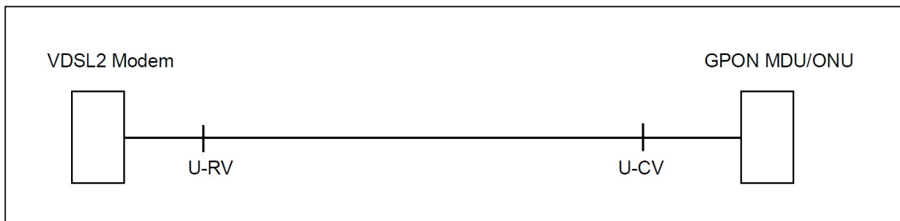
Abbildung Schematische Darstellung eines VDSL2 FTTB Anschluss
